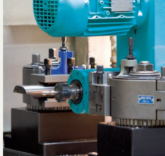
Zylinderbohrung
